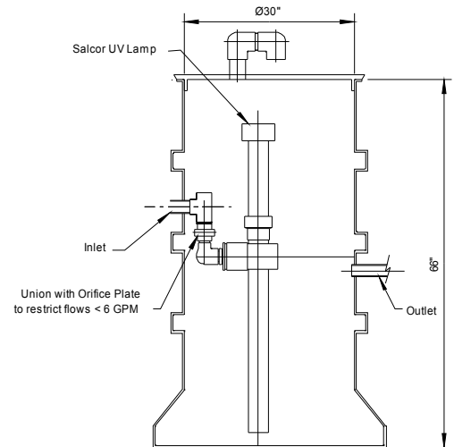
U.V. BASIN
